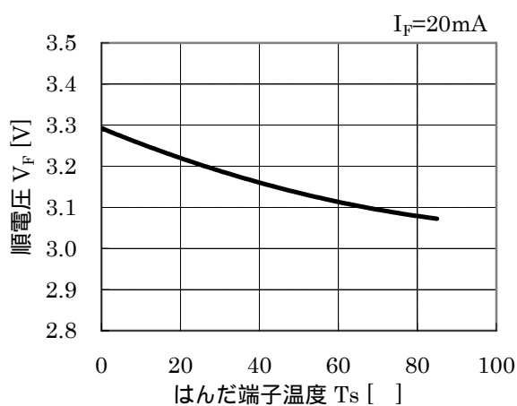
端子温度 順電圧特性
