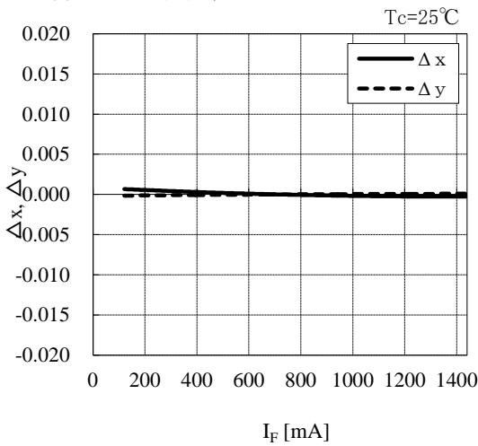
◆順電流－色度変化特性
