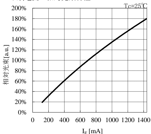
◆順電流－相対光束特性
