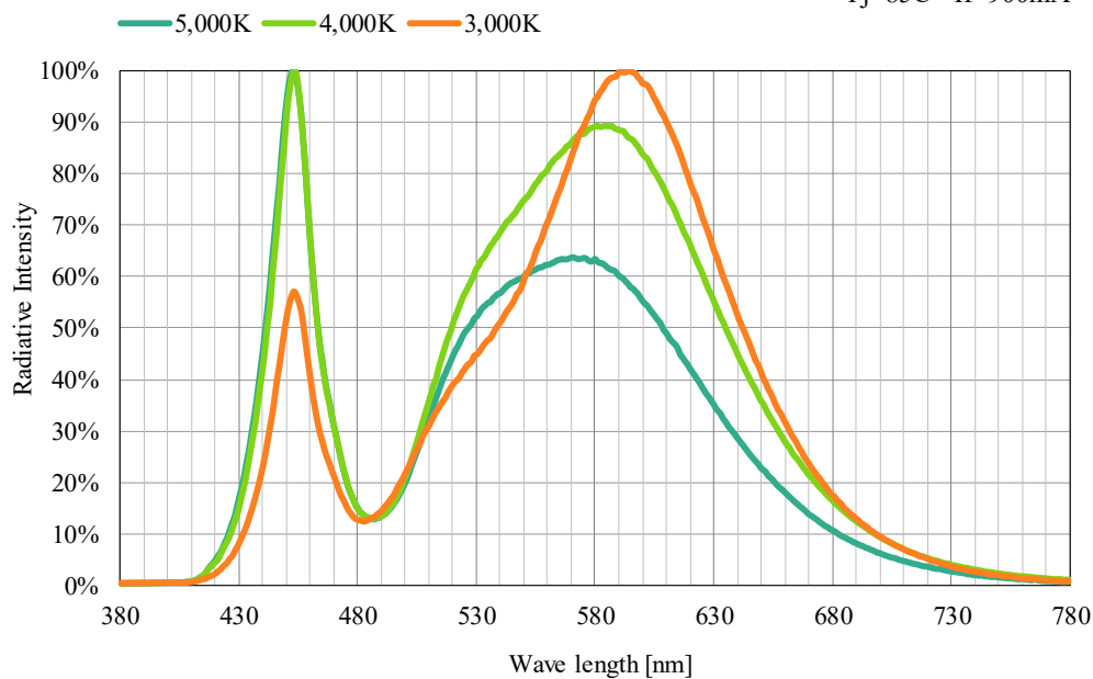
Spectrum : CRI(Ra) 70 Min.
