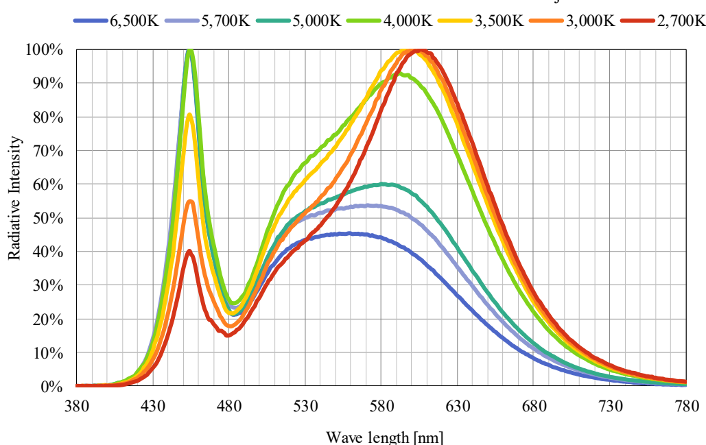
Spectrum : CRI(Ra) 80 Min.
