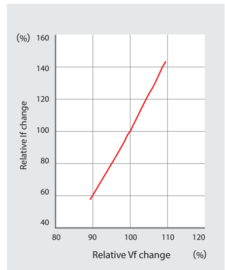
■ 図1 Vf - If characteristic
