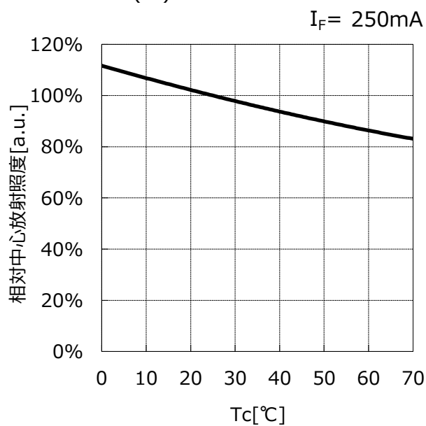
◆ケース温度( T_c )－相対中心放射照度特性
